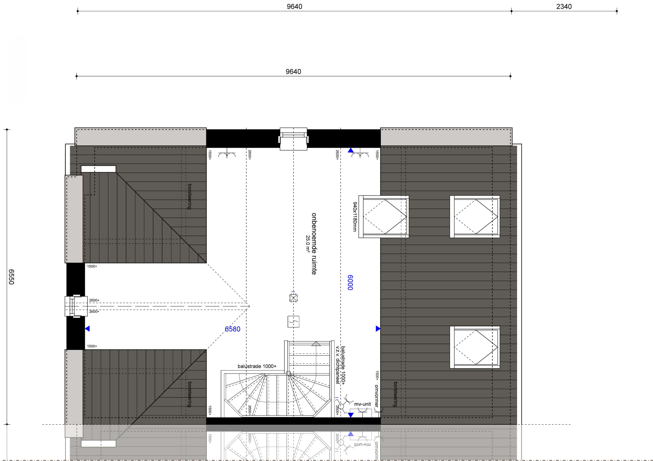
SCHAAL 1 OP 50 Plattegrond ~ Tweede verdieping
